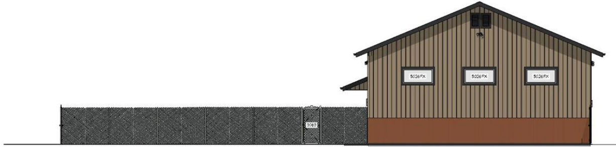
Right Elevation
